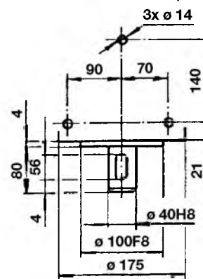
Основная плата - отверстия 3x ø 14
