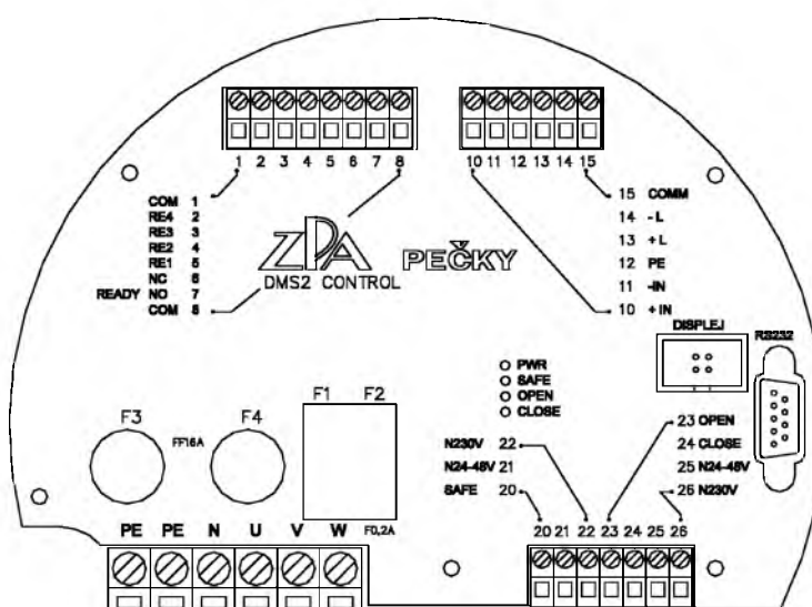
Клеммник DMS2 Аналог
